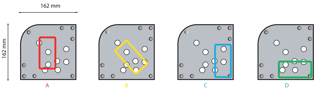
Montageplaat verstelbaar
